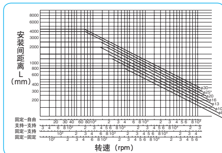
图I-2 危险速度与安装间距离
